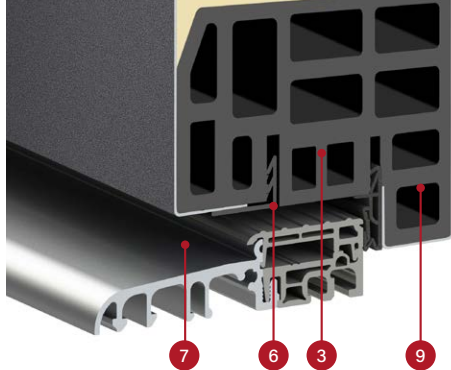
THERMO HOT 78 varčios skerspjūvis su nuleidžiamuoju slenksčiu ir be jo, aliumininis slenkstis
