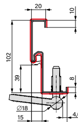
PLIENINĖ KAMPINĖ STAKTA
