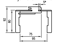
Pjūvis ORB 075
