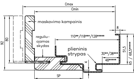
Staktos profilis
