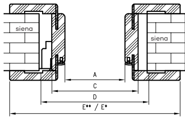
Horizontalus pjūvis OR/ORC
