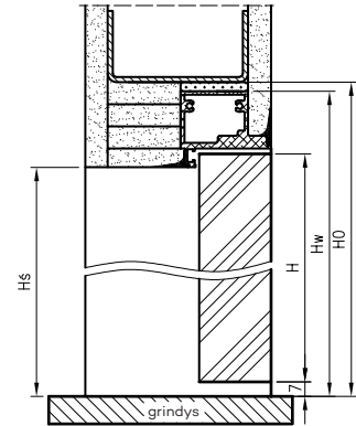
DRE profilis į išorę atsidarančioms lygiabriaunėms durims
