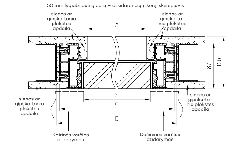
„Profi“ durų pločio matmenys
