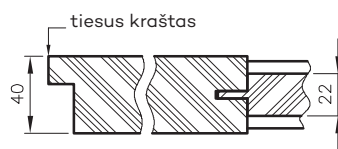
Horizontalus Elsa durų pjūvis
