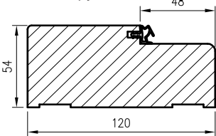
OLIMP EI60 durų medinio staktos pjūvis
