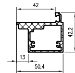
DRE profilis į išorę atsidarančioms lygiabriaunėms durims
