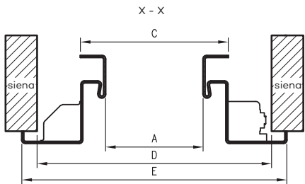
D – angos sienoje plotis
