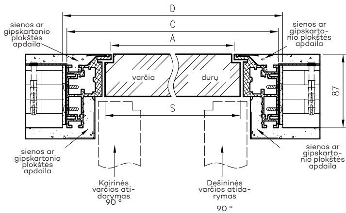
„Profi“ durų pločio matmenys
