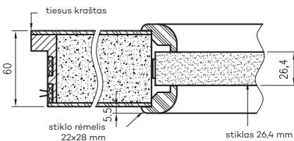
Olimp EI60 ugniai priešgaisrinė durų varčia
