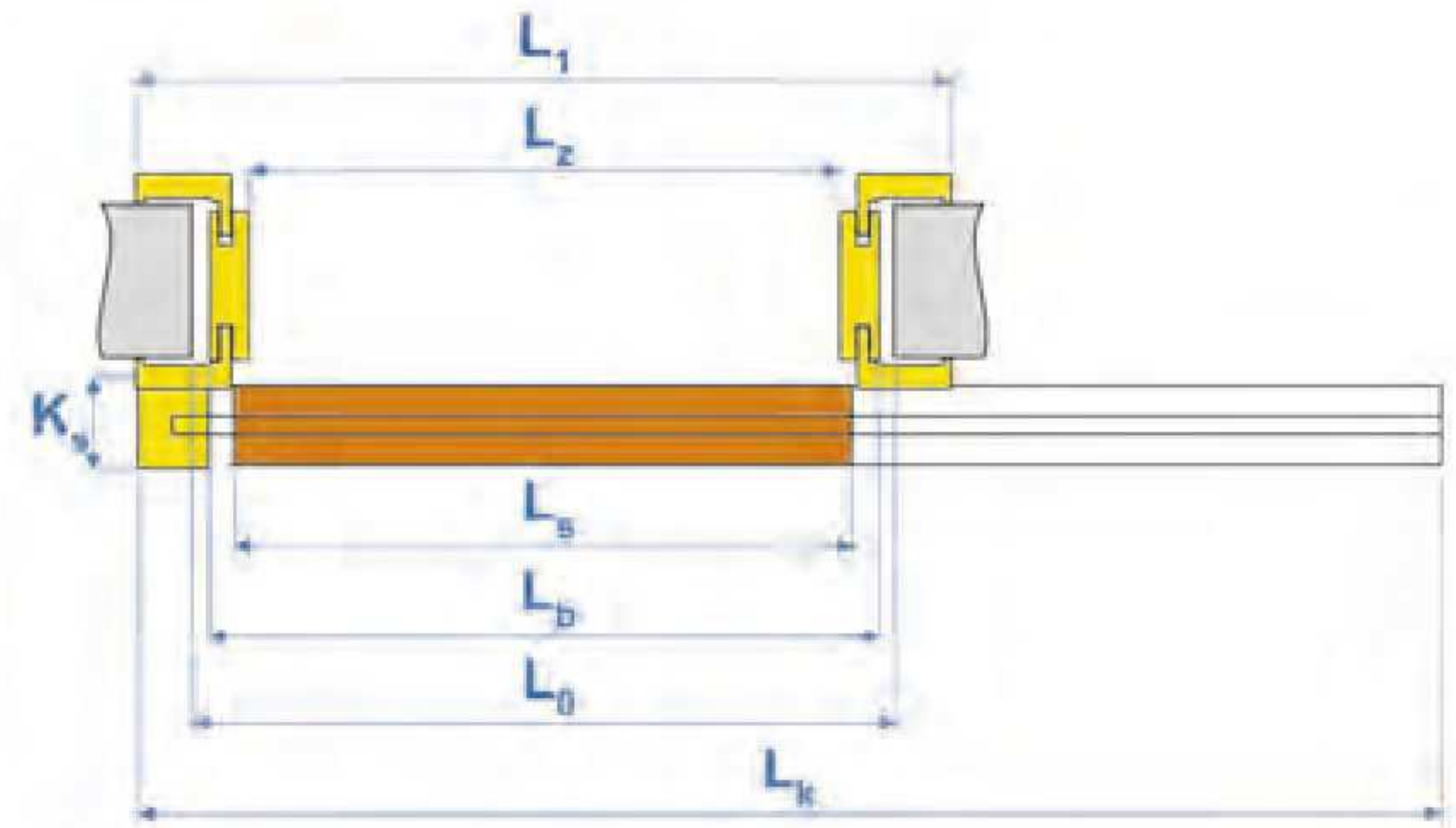
РОЗСУВНА СИСТЕМА З КОРОБКОЮ ECO-SLIDE З КОРОБКОЮ ECO-FIT
